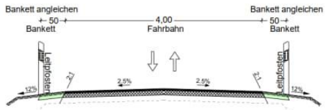
K18 Schnitt I Bau-km ~0+003 - 1+287
